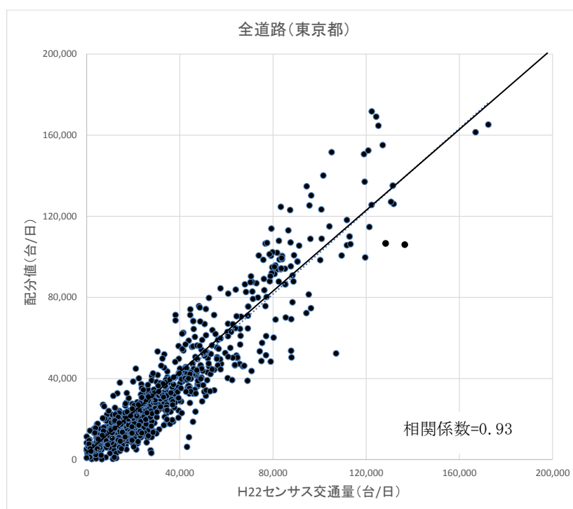
図 2.3-1 交通量の実績値と推計値(全道路：東京都)
